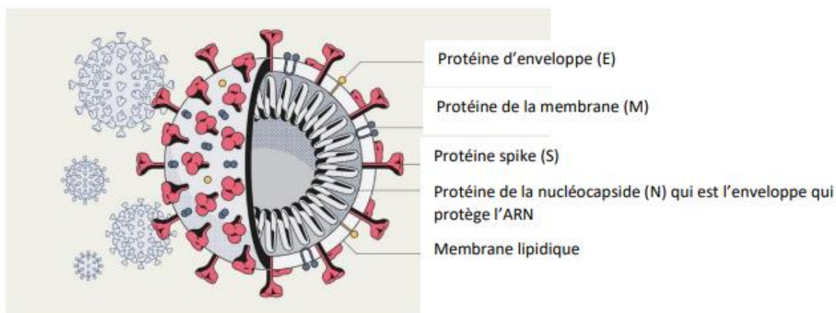
Figure 2 : représentation schématique du coronavirus SARS-Cov-2 (crédit Manuel Bortoletti)
